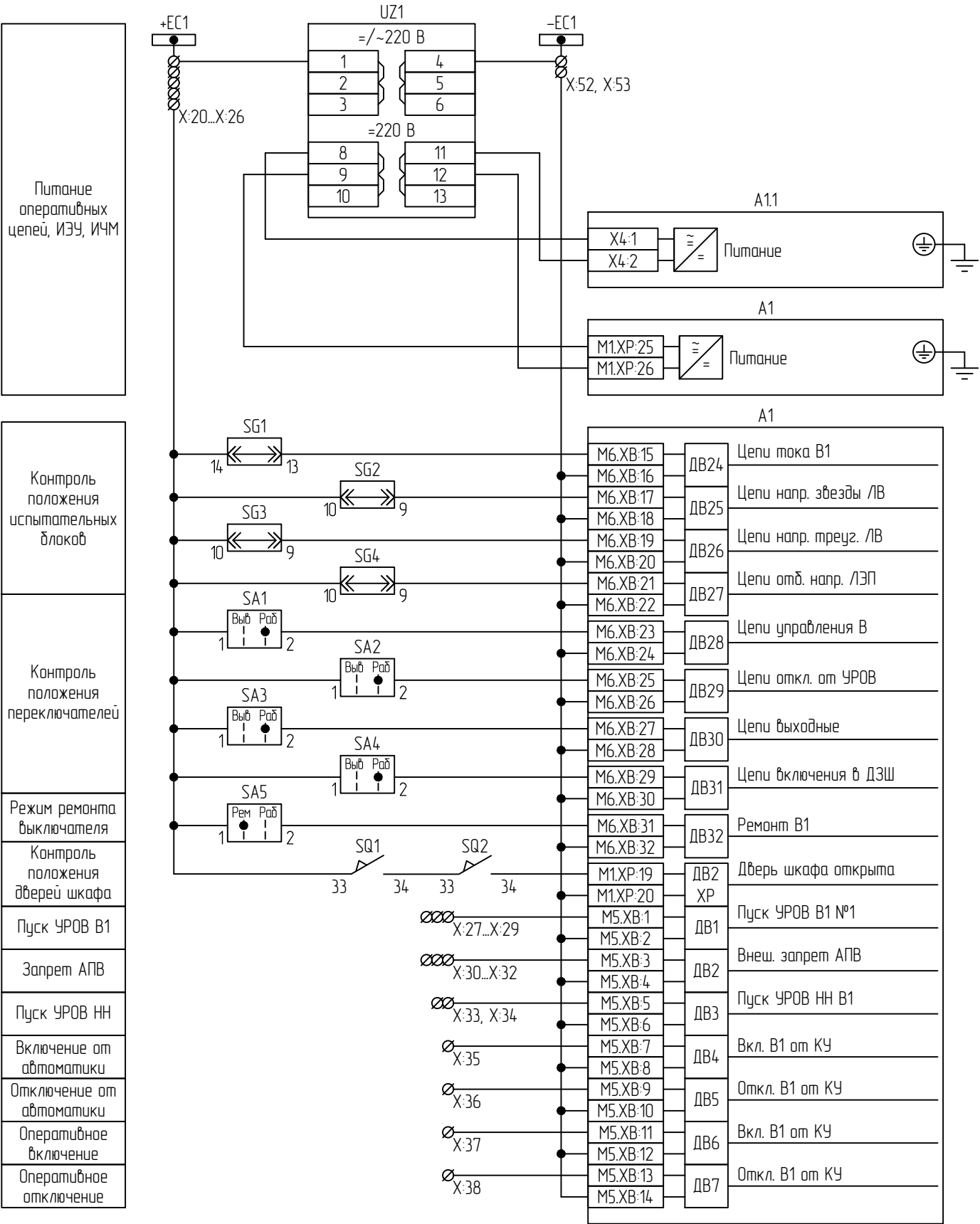
Цепи оперативного тока
